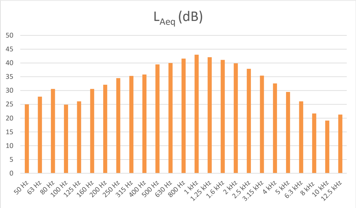
Figura 10 - Espectro relativo à medição 1 de Ruído Ambiente no Ponto R2 para o período diurno (07h-20h)
