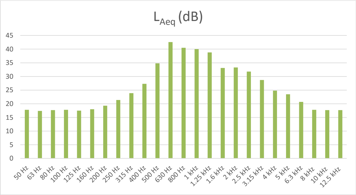
Figura 25 - Espectro relativo à medição 1 de Ruído Ambiente no Ponto R3 para o período noturno (20h-23h)
