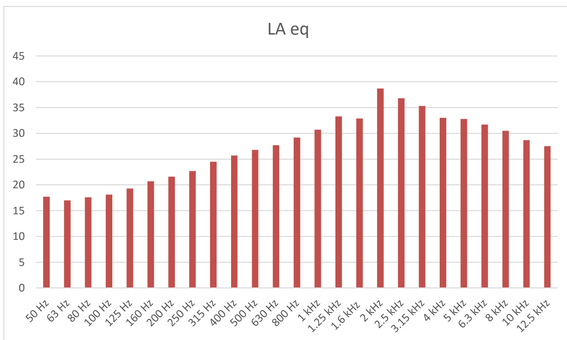
Figura 35 - Espectro relativo à medição 2 de Ruído Ambiente no Ponto R4 para o período noturno (23h-07h)
