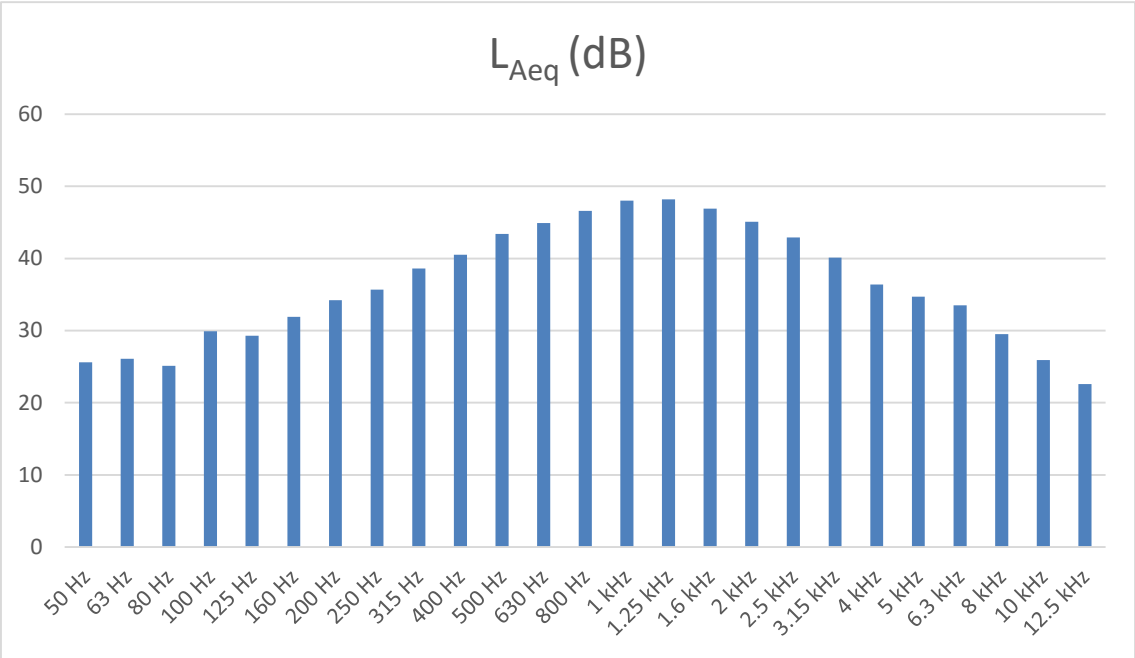
Figura 5 – Espectro da medição 2 relativo às medições de Ruído Ambiente no Ponto R1 para o período entardecer (20h-23h)
