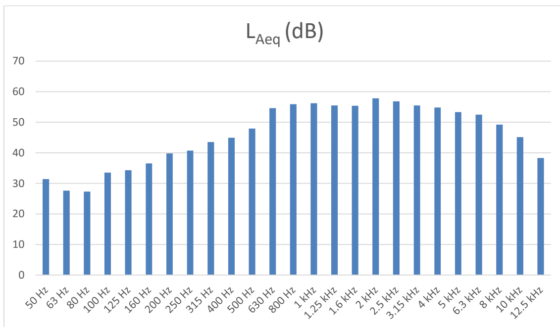
Figura 4 – Espectro da medição 1 relativo às medições de Ruído Ambiente no Ponto R1 para o período entardecer (20h-23h)
