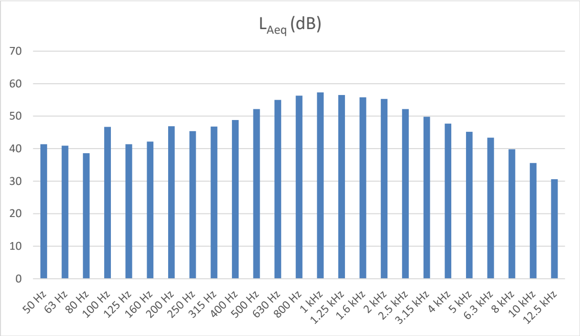
Figura 1 – Espectro da medição 1 relativo às medições de Ruído Ambiente no Ponto R1 para o período diurno (07h-20h)
