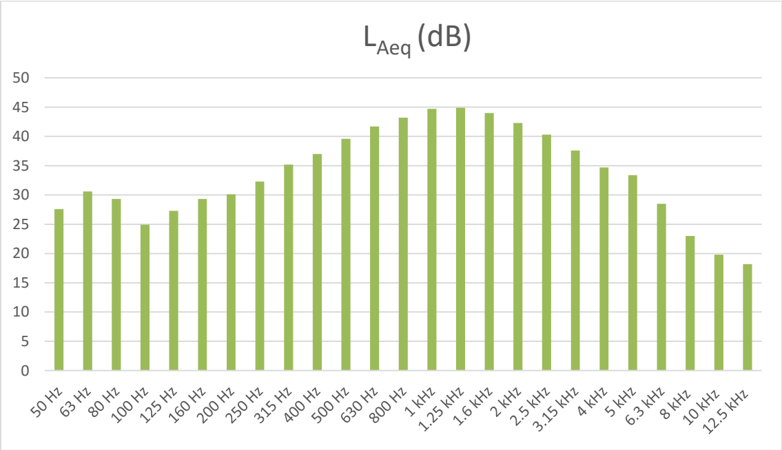
Figura 19 - Espectro relativo à medição 1 de Ruído Ambiente no Ponto R3 para o período diurno (07h-20h)
