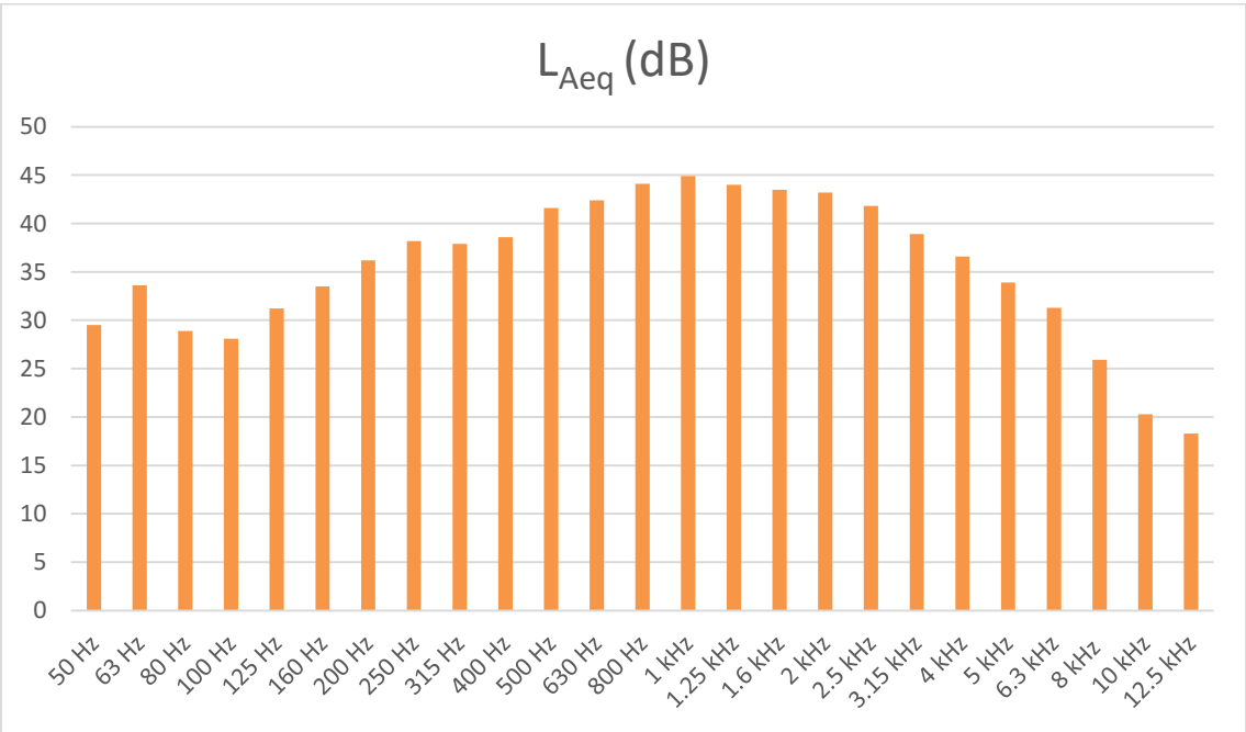
Figura 11 - Espectro relativo à medição 2 de Ruído Ambiente no Ponto R2 para o período diurno (07h-20h)
