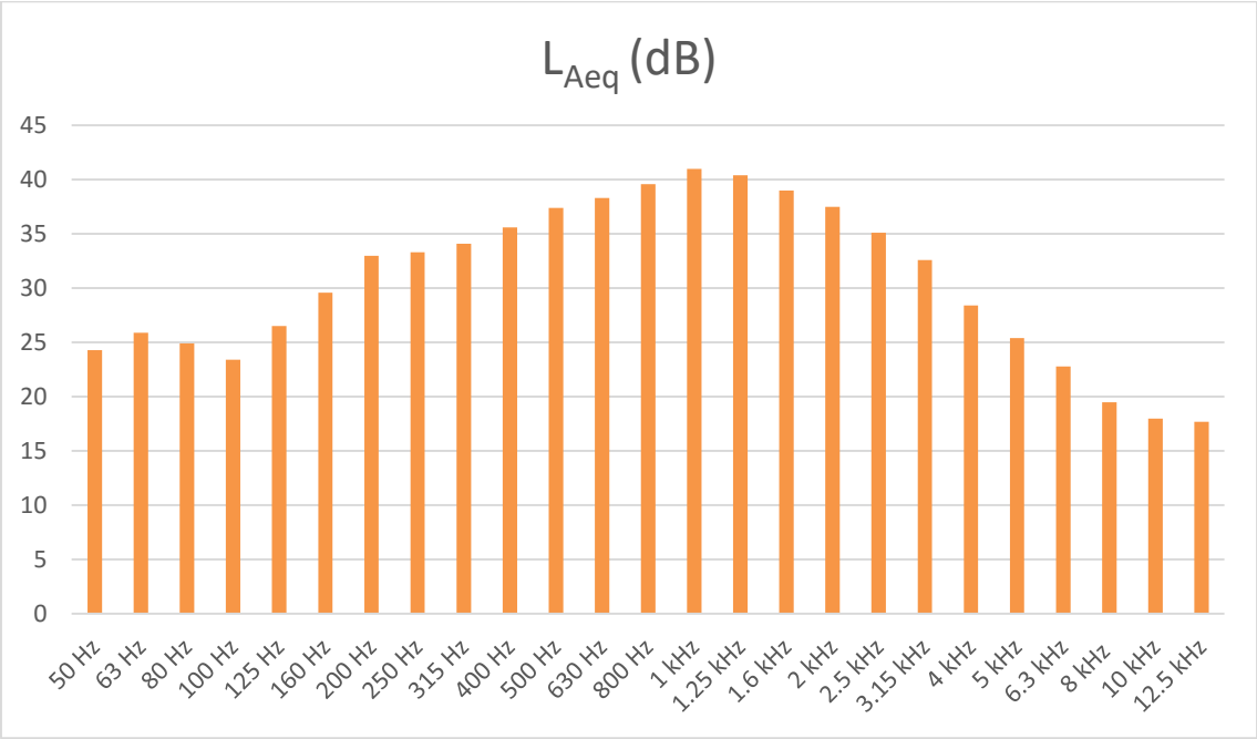
Figura 14 – Espectro da medição 2 relativo às medições de Ruído Ambiente no Ponto R2 para o período entardecer (20h-23h)
