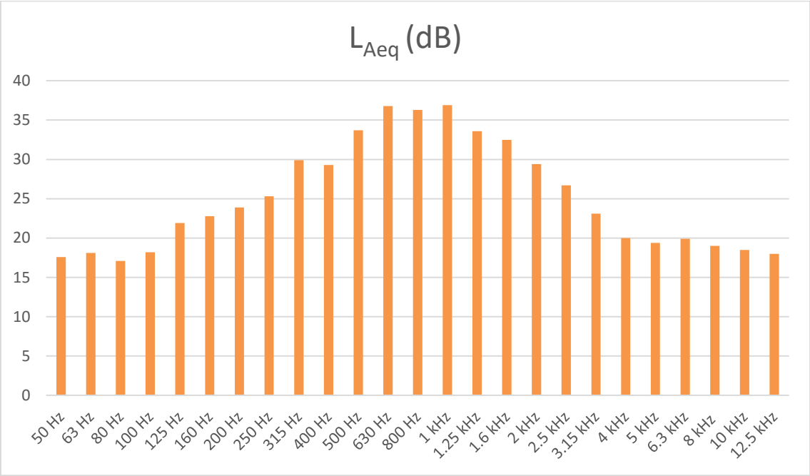
Figura 17 – Espectro da medição 2 relativo às medições de Ruído Ambiente no Ponto R2 para o período noturno (23h-07h)
