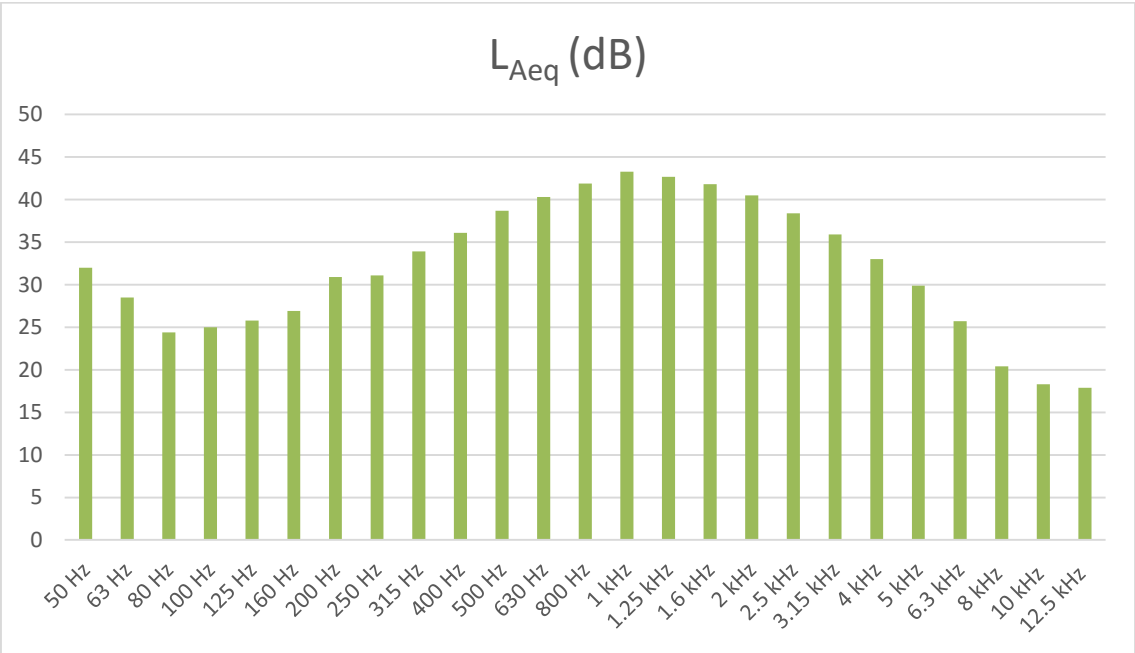
Figura 20 - Espectro relativo à medição 2 de Ruído Ambiente no Ponto R3 para o período diurno (07h-20h)
