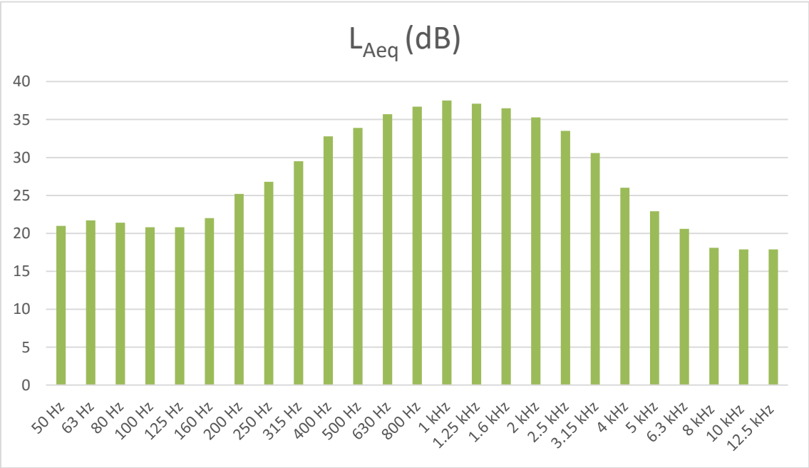
Figura 24 - Espectro relativo à medição 3 de Ruído Ambiente no Ponto R3 para o período entardecer (20h-23h)
