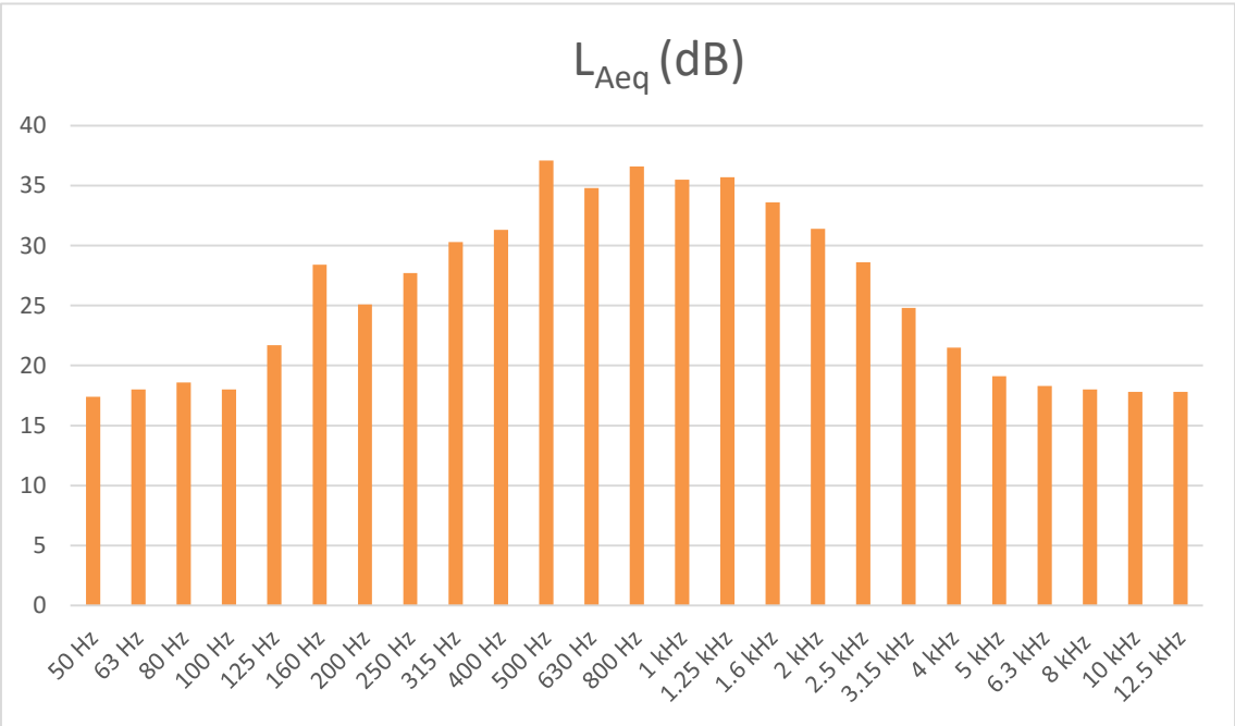
Figura 15 – Espectro da medição 3 relativo às medições de Ruído Ambiente no Ponto R2 para o período entardecer (20h-23h)
