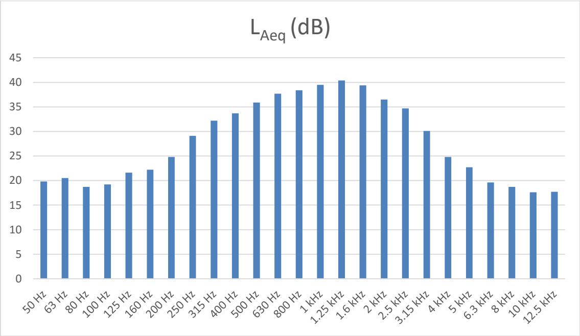
Figura 9 – Espectro da medição 3 relativo às medições de Ruído Ambiente no Ponto R1 para o período noturno (23h-07h)
