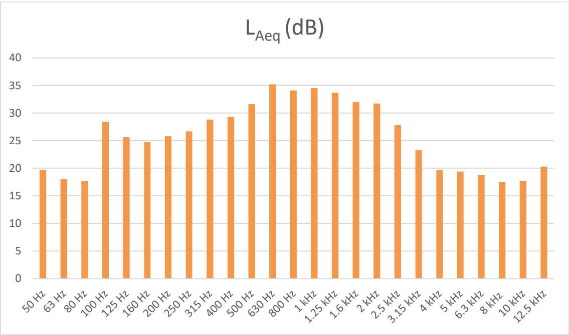
Figura 18 – Espectro da medição 3 relativo às medições de Ruído Ambiente no Ponto R2 para o período noturno (23h-07h)
