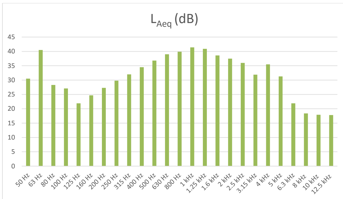
Figura 21 - Espectro relativo à medição 3 de Ruído Ambiente no Ponto R3 para o período diurno (07h-20h)
