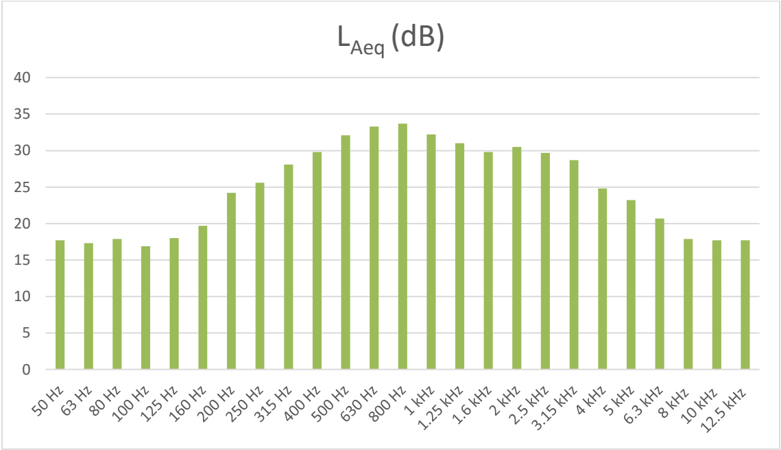
Figura 27 - Espectro relativo à medição 3 de Ruído Ambiente no Ponto R3 para o período noturno (20h-23h)
