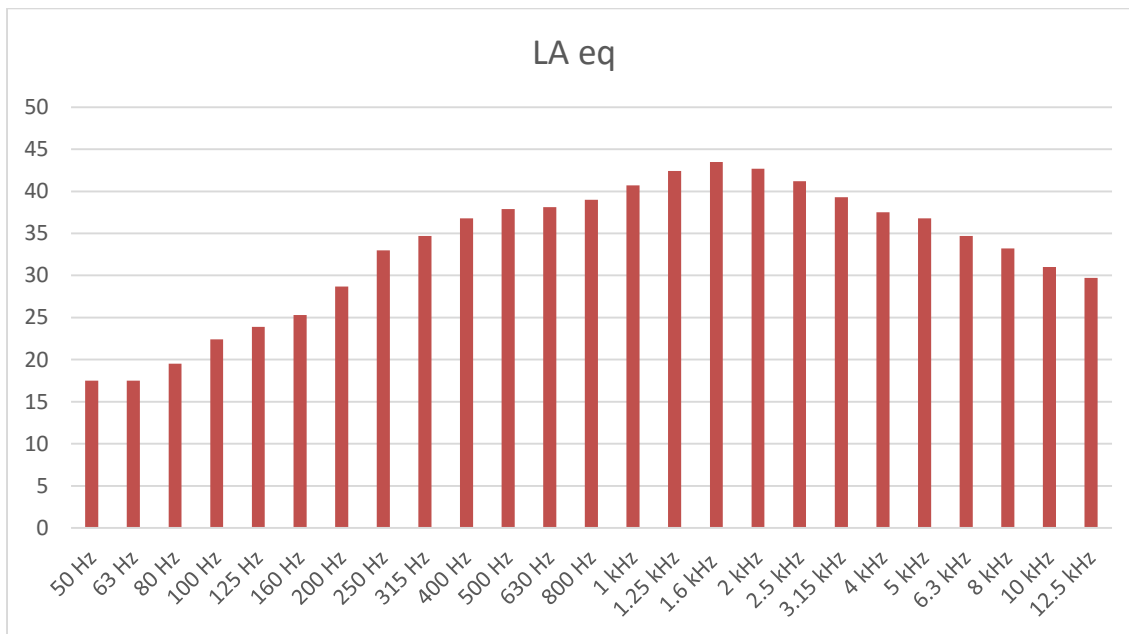
Figura 31 - Espectro relativo à medição 1 de Ruído Ambiente no Ponto R4 para o período entardecer (20h-23h)
