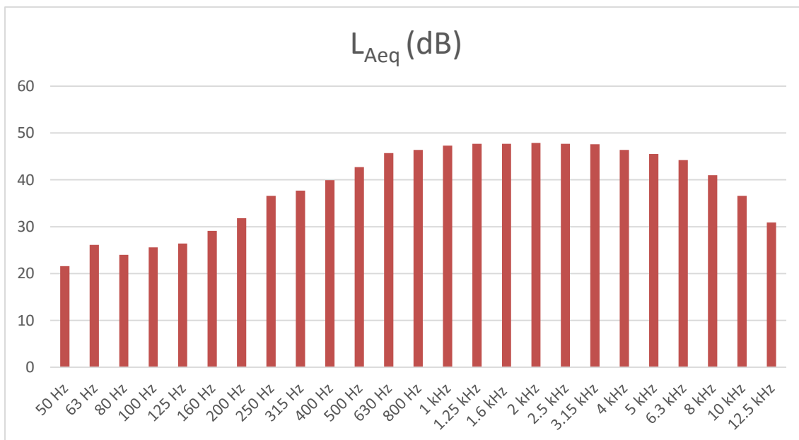
Figura 29 - Espectro relativo à medição 2 de Ruído Ambiente no Ponto R4 para o período diurno (07h-20h)
