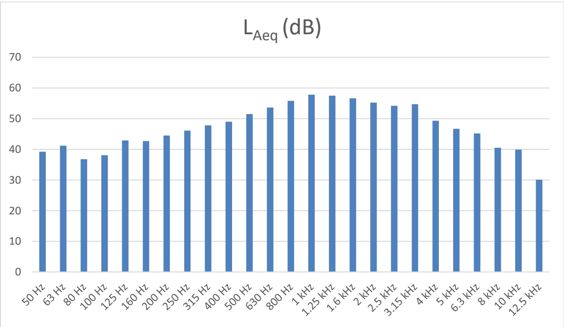
Figura 2 – Espectro da medição 2 relativo às medições de Ruído Ambiente no Ponto R1 para o período diurno (07h-20h)
