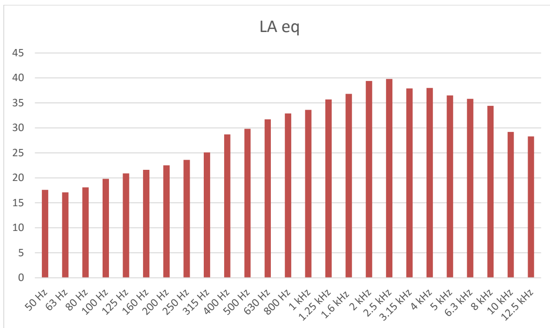
Figura 34 - Espectro relativo à medição 1 de Ruído Ambiente no Ponto R4 para o período noturno (23h-07h)
