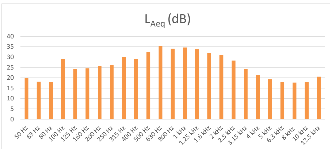
Figura 16 – Espectro da medição 1 relativo às medições de Ruído Ambiente no Ponto R2 para o período noturno (23h-07h)
