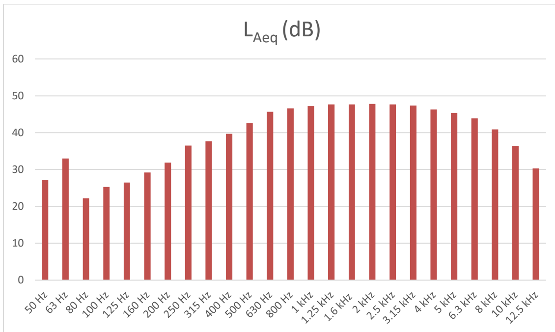
Figura 28 - Espectro relativo à medição 1 de Ruído Ambiente no Ponto R4 para o período diurno (07h-20h)
