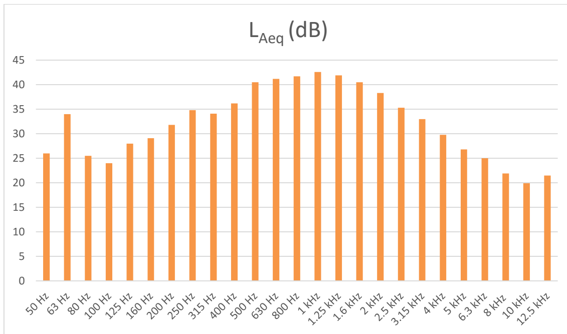
Figura 12 - Espectro relativo à medição 3 de Ruído Ambiente no Ponto R2 para o período diurno (07h-20h)
