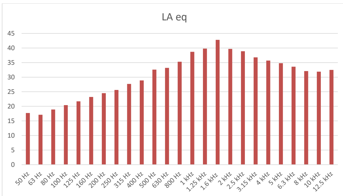
Figura 32 - Espectro relativo à medição 2 de Ruído Ambiente no Ponto R4 para o período entardecer (20h-23h)
