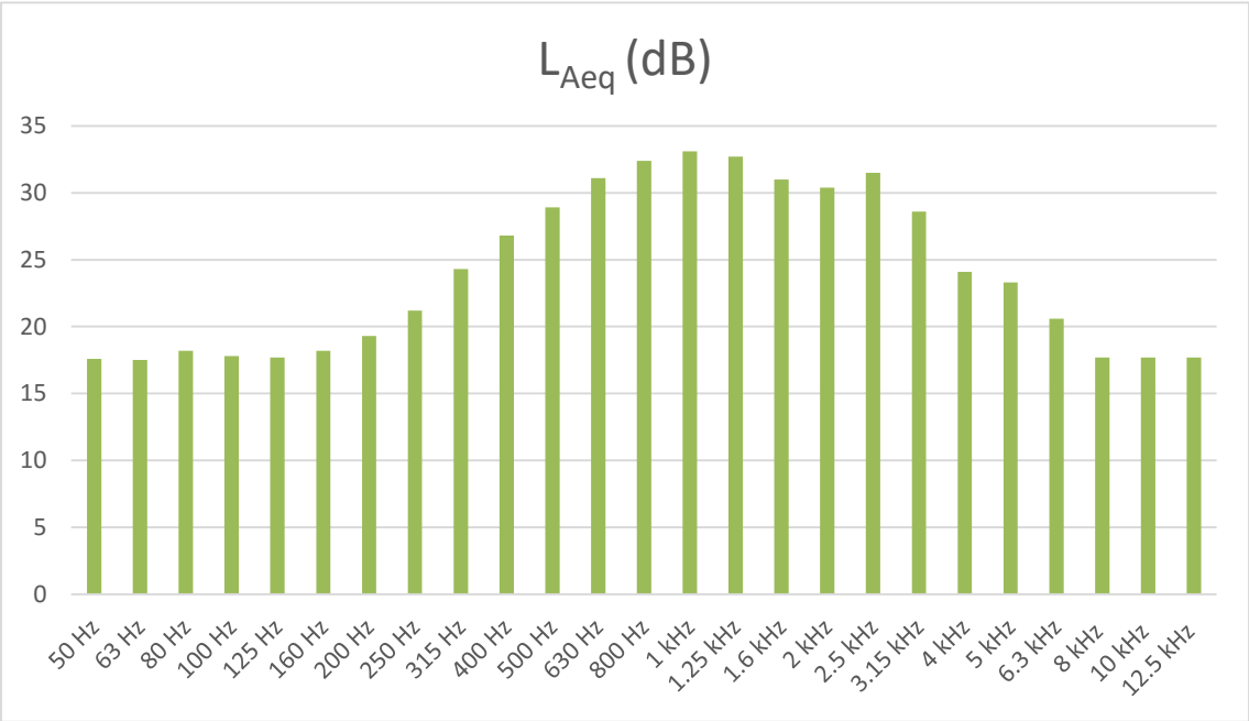
Figura 25 - Espectro relativo à medição 1 de Ruído Ambiente no Ponto R3 para o período noturno (20h-23h)
