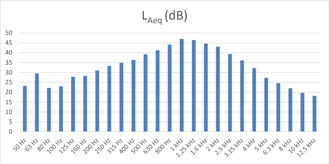
Figura 7 – Espectro da medição 1 relativo às medições de Ruído Ambiente no Ponto R1 para o período noturno (23h-07h)
