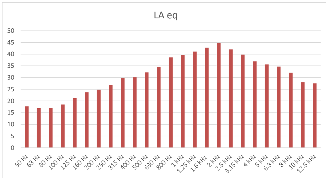
Figura 33 - Espectro relativo à medição 3 de Ruído Ambiente no Ponto R4 para o período entardecer (20h-23h)
