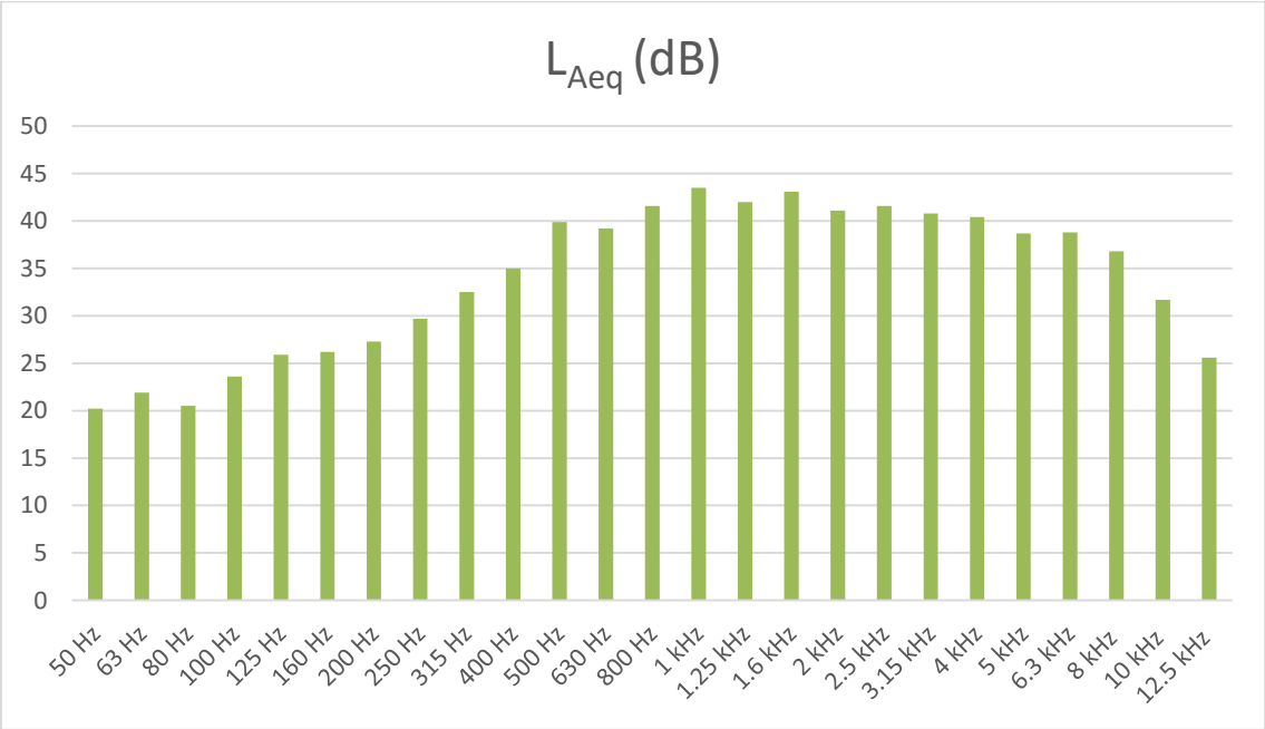
Figura 23 - Espectro relativo à medição 2 de Ruído Ambiente no Ponto R3 para o período entardecer (20h-23h)
