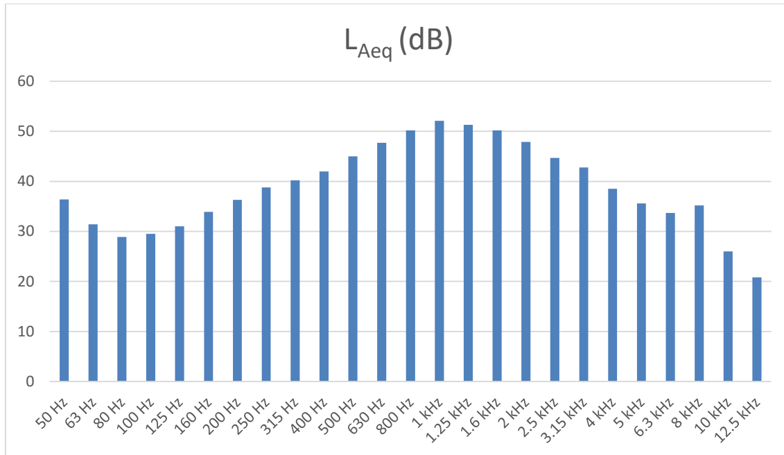
Figura 3 – Espectro da medição 3 relativo às medições de Ruído Ambiente no Ponto R1 para o período diurno (07h-20h)
